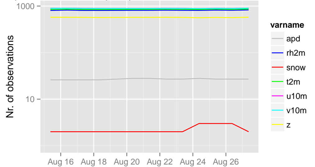
/opdata/arome2_5_preop/ecma_sfc/ts/ecma.db 09 UTC
