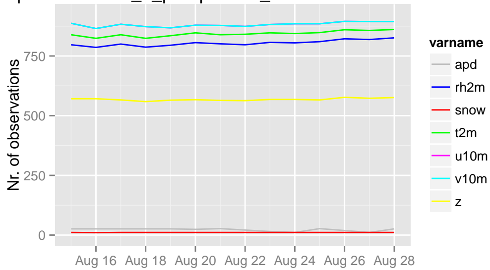
/opdata/arome2_5_preop/ecma_sfc/ts/ecma.db 00 UTC
