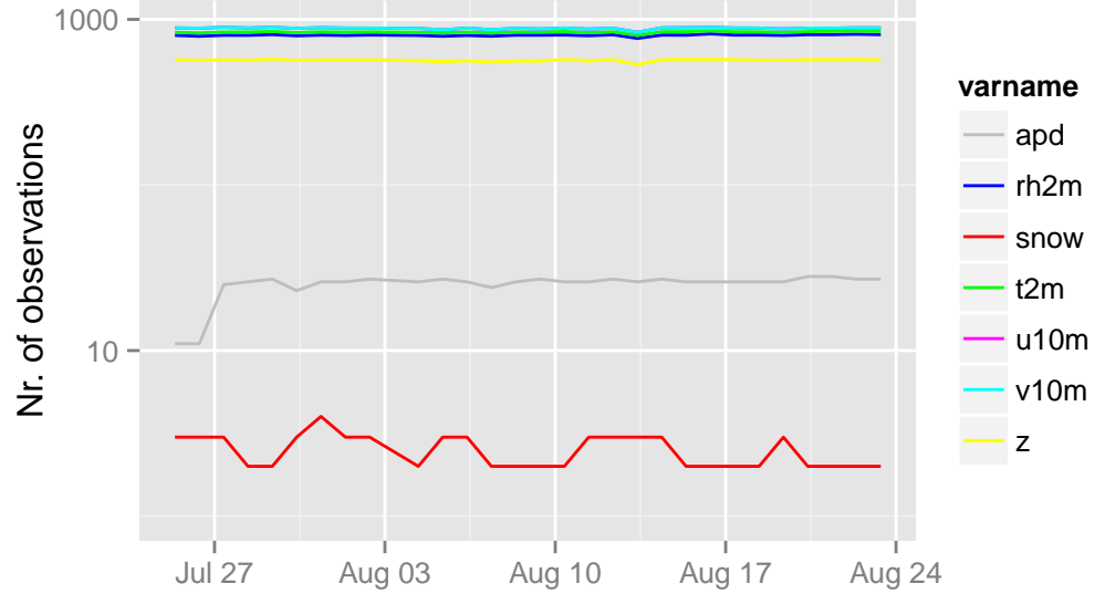
/opdata/arome2_5_main/ecma_sfc/ts/ecma.db 09 UTC
