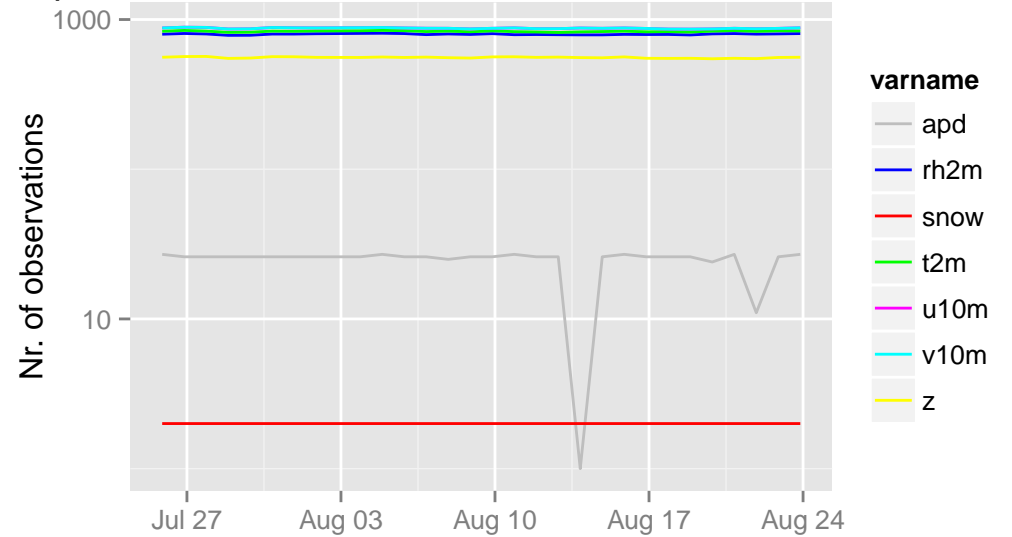
/opdata/arome2_5_main/ecma_sfc/ts/ecma.db 21 UTC
