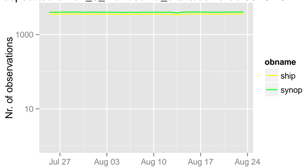
/opdata/arome2_5_main/ecma_sfc/ts/ecma.db 09 UTC
