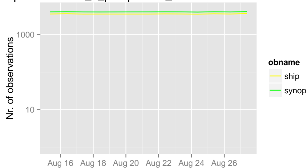
/opdata/arome2_5_preop/ecma_sfc/ts/ecma.db 09 UTC
