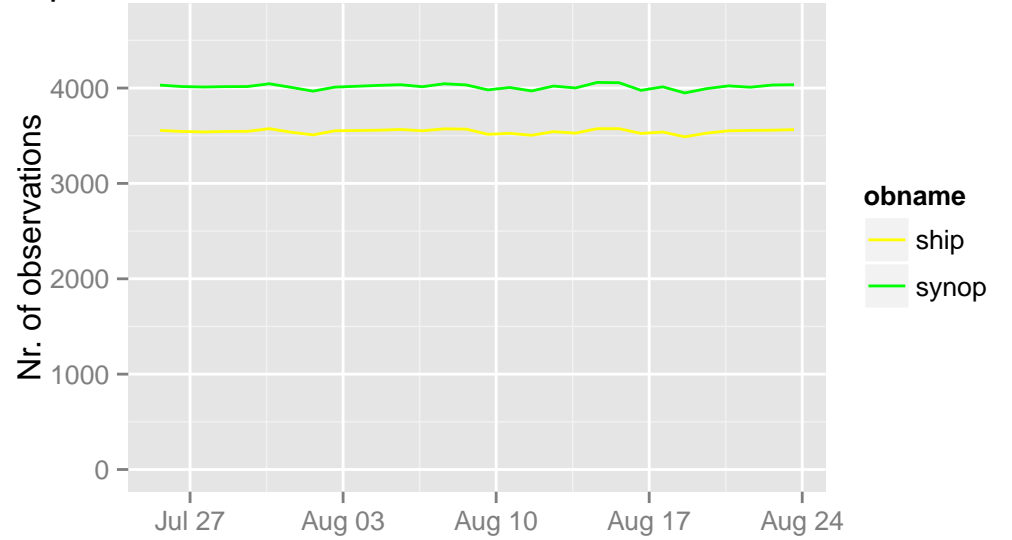
/opdata/arome2_5_main/ecma_sfc/ts/ecma.db 15 UTC
