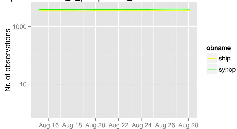
/opdata/arome2_5_preop/ecma_sfc/ts/ecma.db 03 UTC
