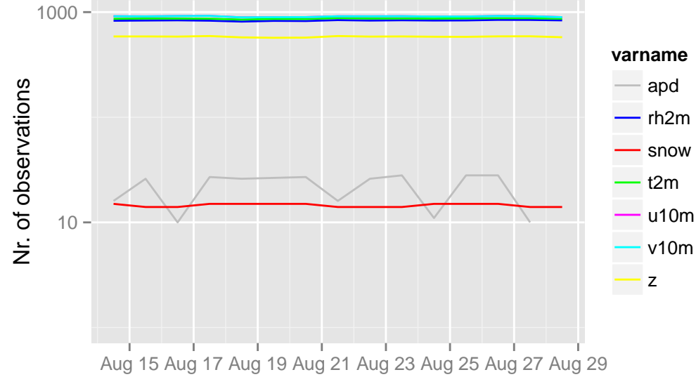
/opdata/arome2_5_preop/ecma_sfc/ts/ecma.db 12 UTC
