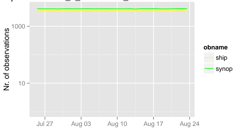
/opdata/arome2_5_main/ecma_sfc/ts/ecma.db 12 UTC
