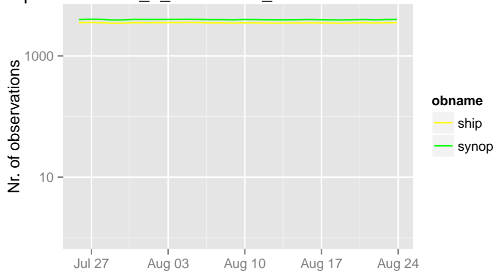
/opdata/arome2_5_main/ecma_sfc/ts/ecma.db 21 UTC
