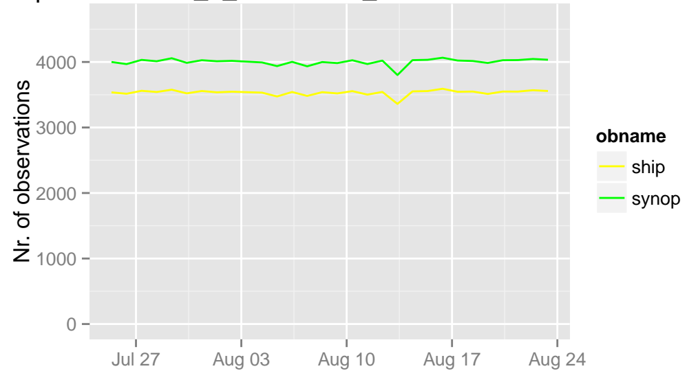
/opdata/arome2_5_main/ecma_sfc/ts/ecma.db 09 UTC
