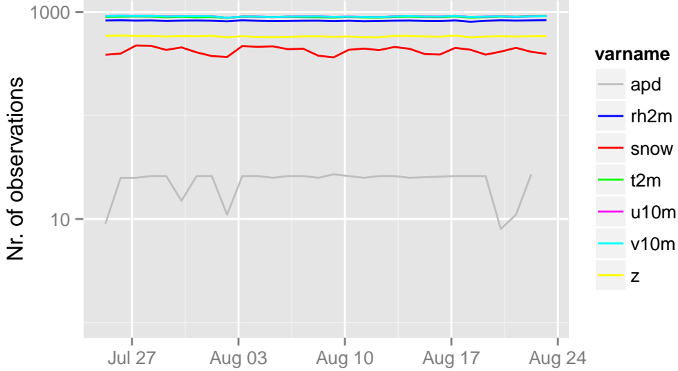
/opdata/arome2_5_main/ecma_sfc/ts/ecma.db 06 UTC
