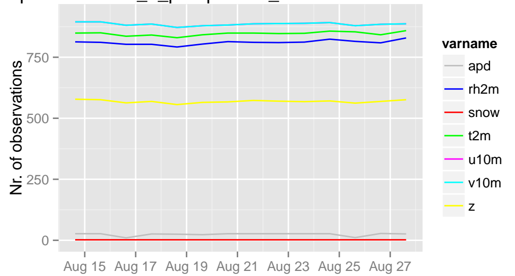
/opdata/arome2_5_preop/ecma_sfc/ts/ecma.db 15 UTC
