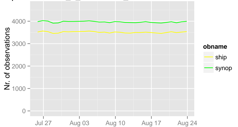
/opdata/arome2_5_main/ecma_sfc/ts/ecma.db 21 UTC
