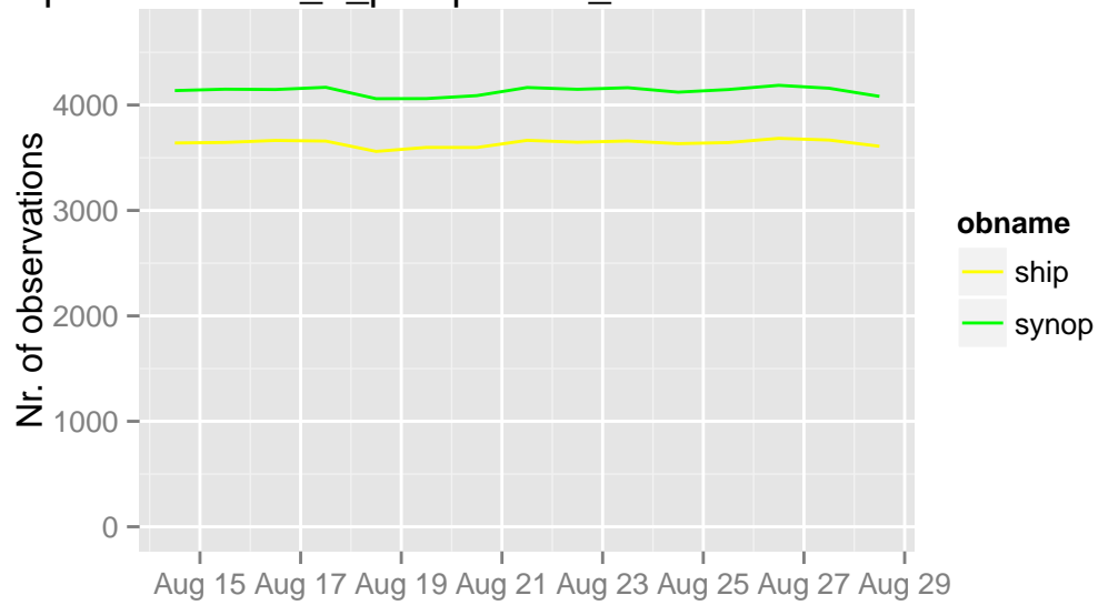
/opdata/arome2_5_preop/ecma_sfc/ts/ecma.db 12 UTC
