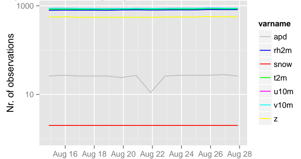
/opdata/arome2_5_preop/ecma_sfc/ts/ecma.db 21 UTC
