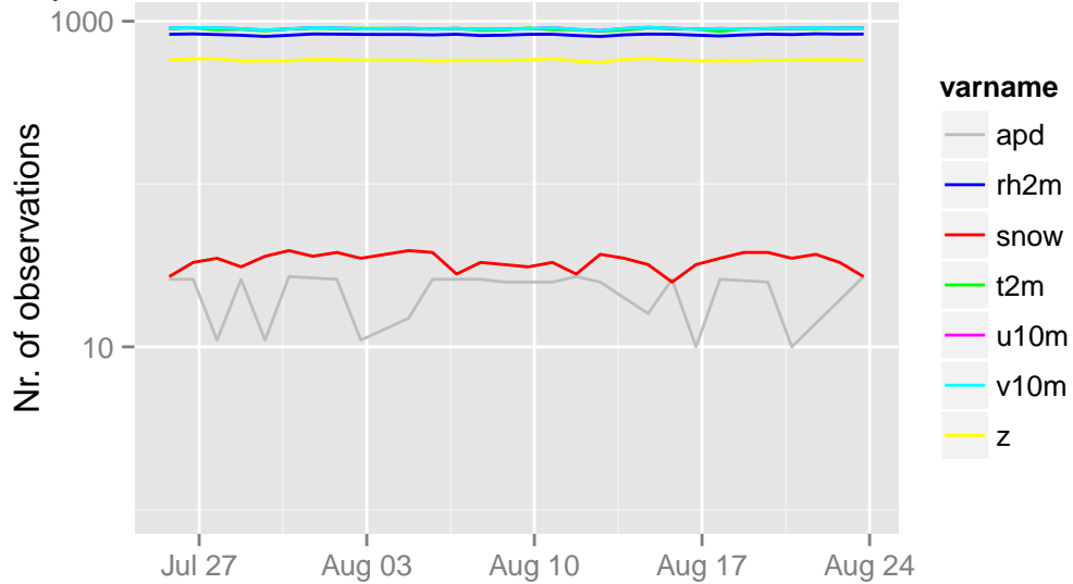
/opdata/arome2_5_main/ecma_sfc/ts/ecma.db 18 UTC
