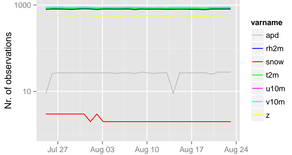
/opdata/arome2_5_main/ecma_sfc/ts/ecma.db 03 UTC
