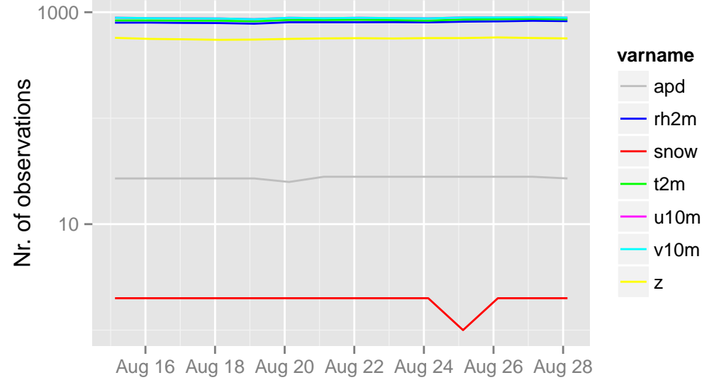
/opdata/arome2_5_preop/ecma_sfc/ts/ecma.db 03 UTC
