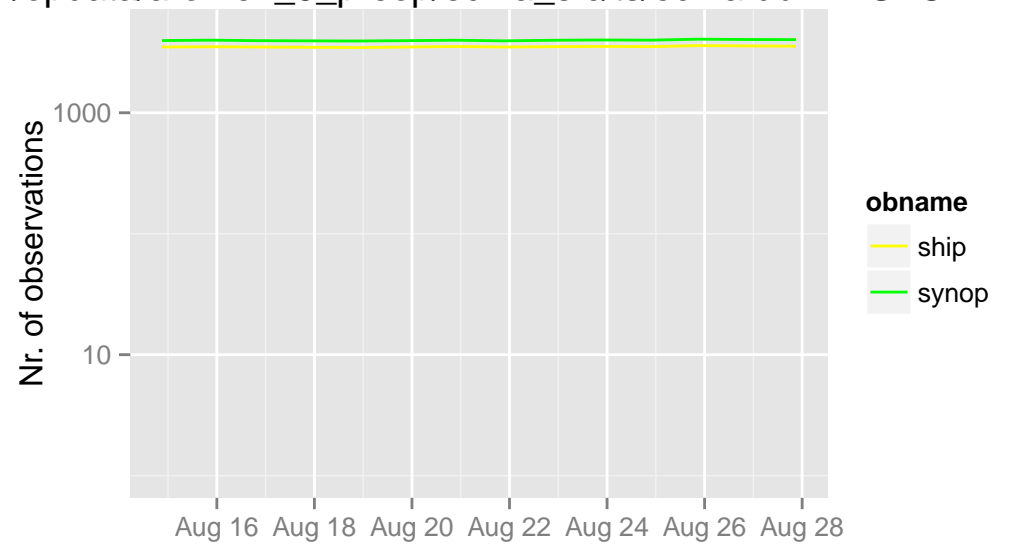
/opdata/arome2_5_preop/ecma_sfc/ts/ecma.db 21 UTC
