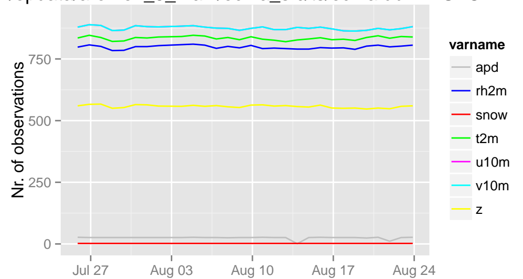
/opdata/arome2_5_main/ecma_sfc/ts/ecma.db 21 UTC
