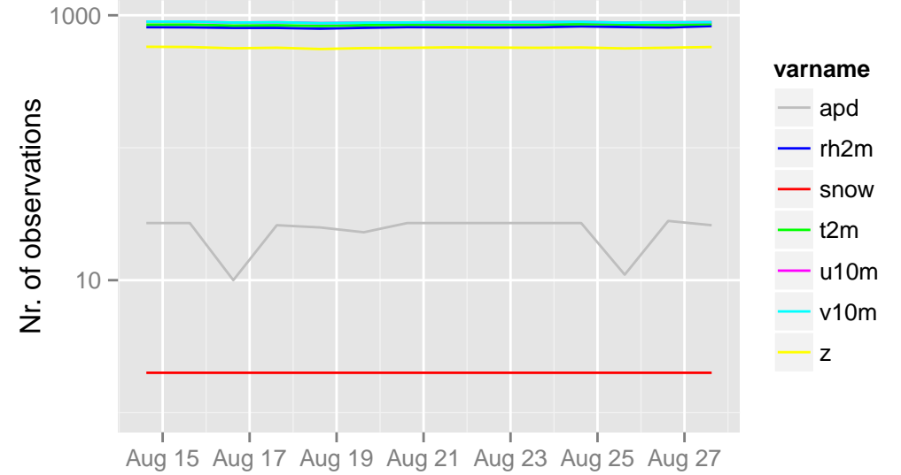
/opdata/arome2_5_preop/ecma_sfc/ts/ecma.db 15 UTC
