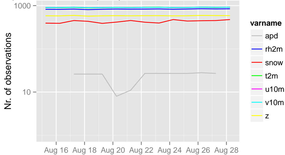
/opdata/arome2_5_preop/ecma_sfc/ts/ecma.db 06 UTC
