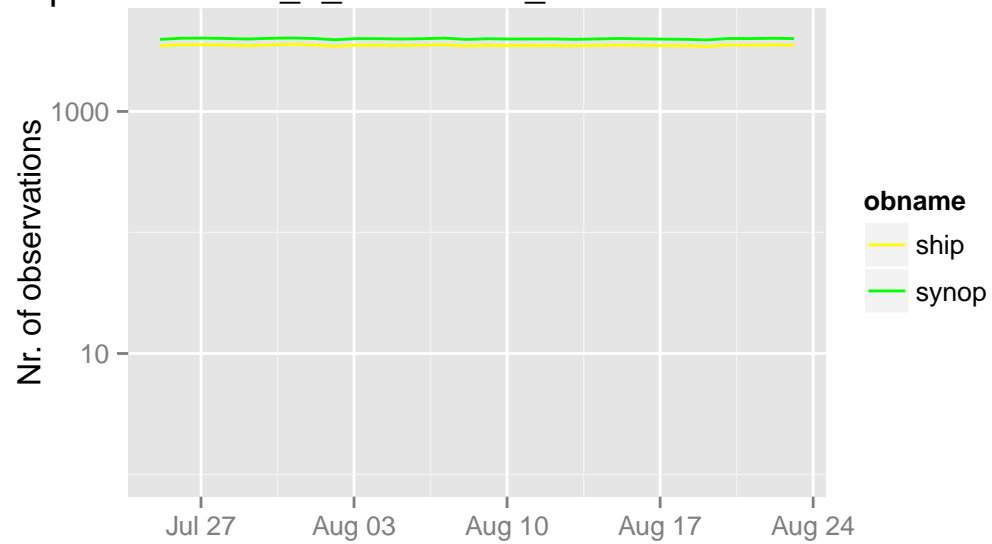
/opdata/arome2_5_main/ecma_sfc/ts/ecma.db 03 UTC
