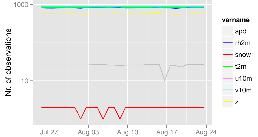
/opdata/arome2_5_main/ecma_sfc/ts/ecma.db 15 UTC
