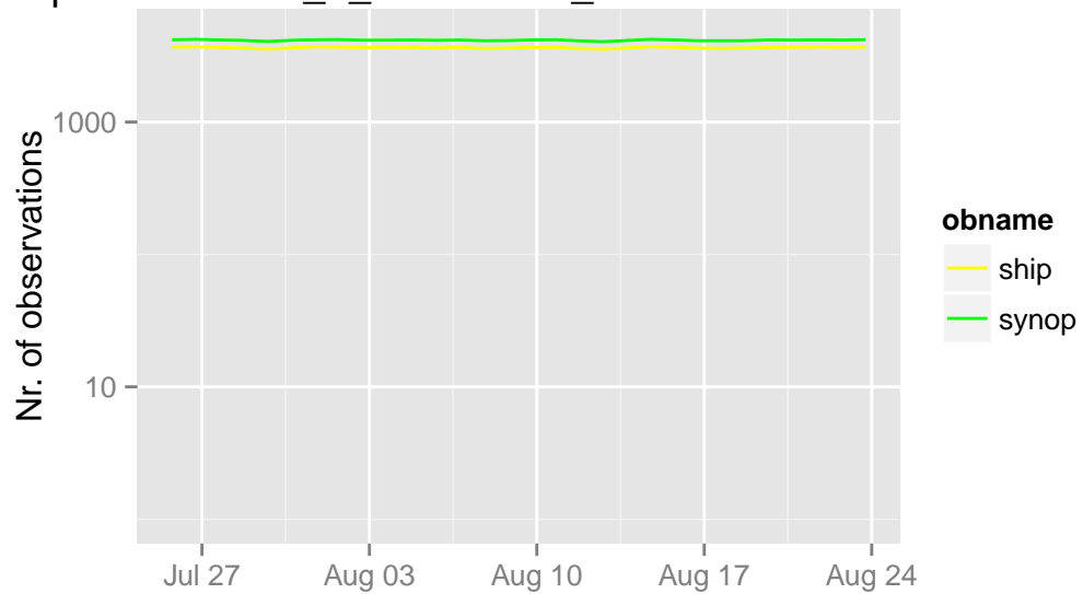
/opdata/arome2_5_main/ecma_sfc/ts/ecma.db 18 UTC
