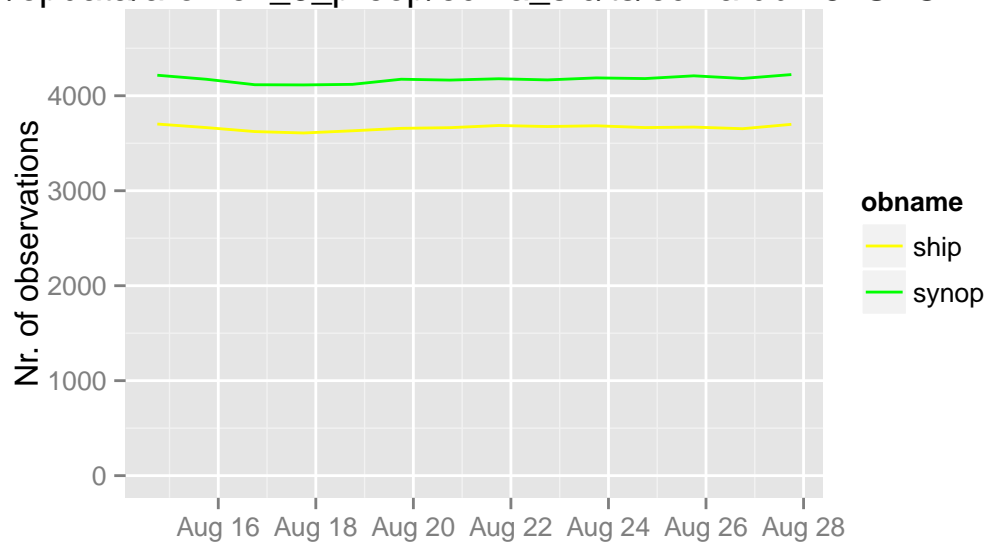
/opdata/arome2_5_preop/ecma_sfc/ts/ecma.db 18 UTC
