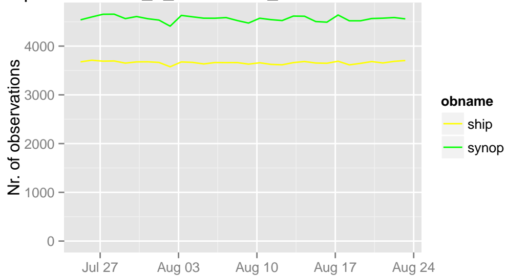
/opdata/arome2_5_main/ecma_sfc/ts/ecma.db 06 UTC
