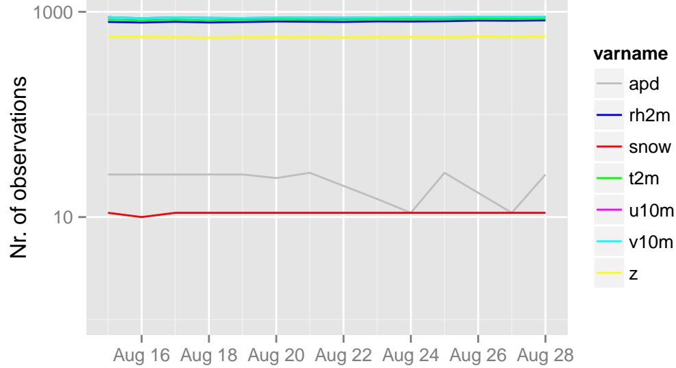
/opdata/arome2_5_preop/ecma_sfc/ts/ecma.db 00 UTC
