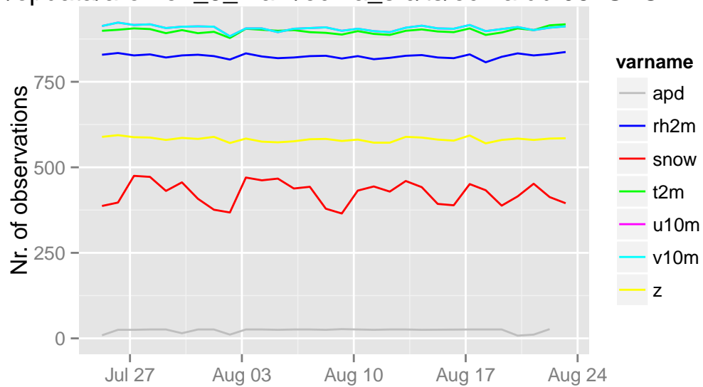
/opdata/arome2_5_main/ecma_sfc/ts/ecma.db 06 UTC
