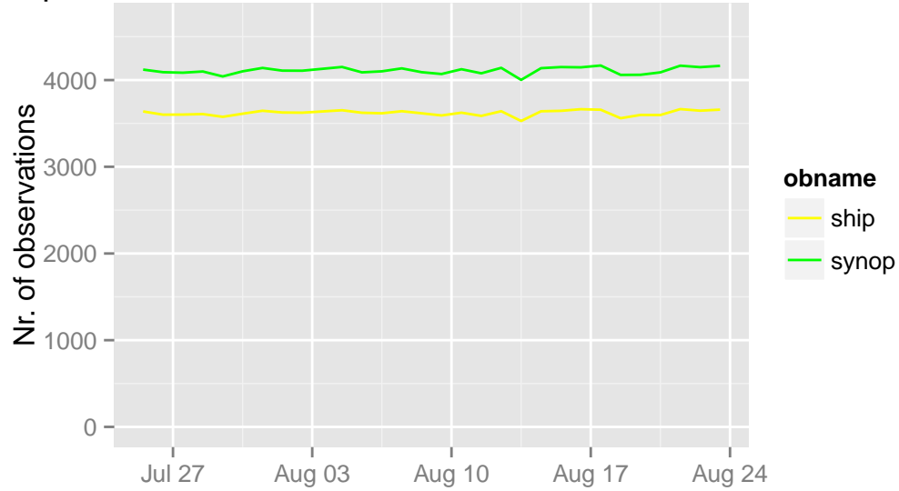
/opdata/arome2_5_main/ecma_sfc/ts/ecma.db 12 UTC
