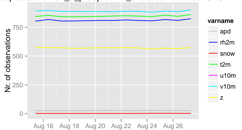
/opdata/arome2_5_preop/ecma_sfc/ts/ecma.db 09 UTC
