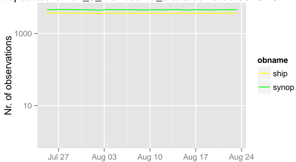
/opdata/arome2_5_main/ecma_sfc/ts/ecma.db 06 UTC
