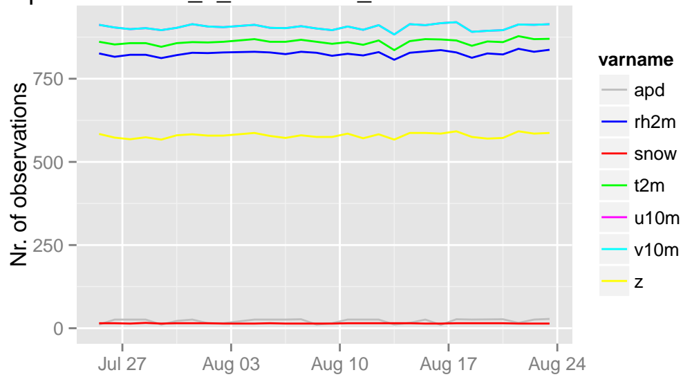
/opdata/arome2_5_main/ecma_sfc/ts/ecma.db 12 UTC
