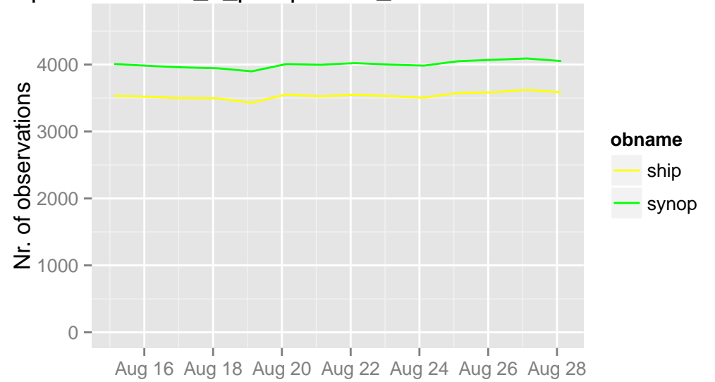
/opdata/arome2_5_preop/ecma_sfc/ts/ecma.db 03 UTC
