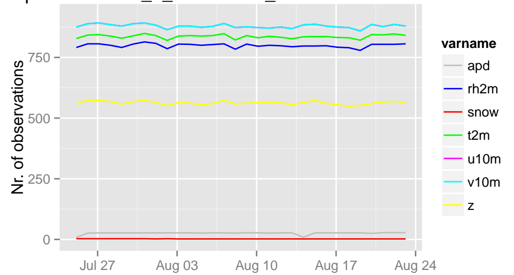
/opdata/arome2_5_main/ecma_sfc/ts/ecma.db 03 UTC
