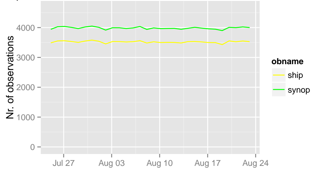
/opdata/arome2_5_main/ecma_sfc/ts/ecma.db 03 UTC
