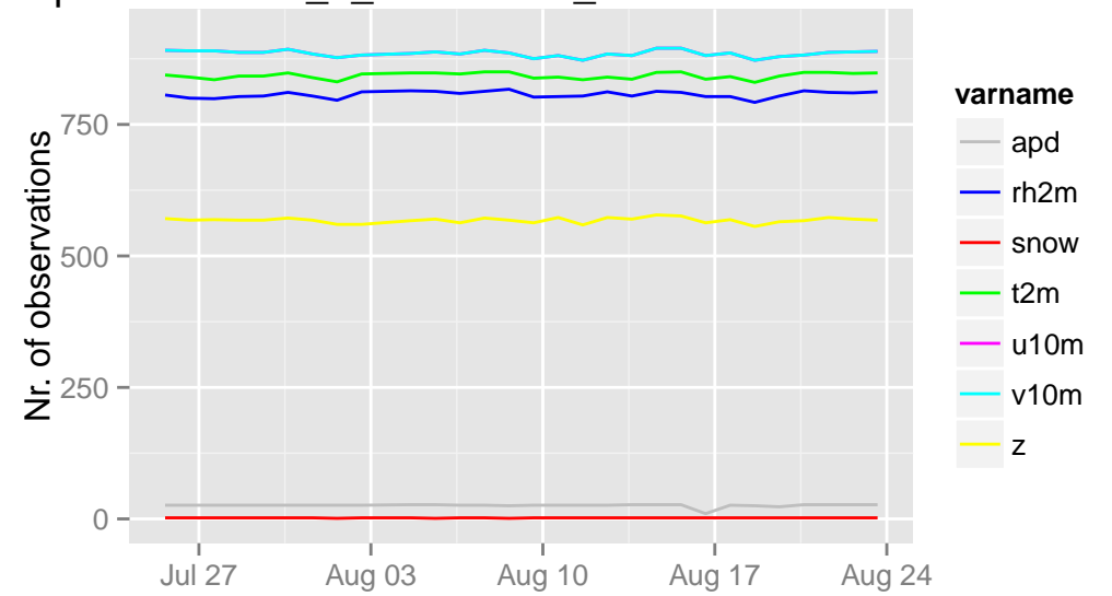
/opdata/arome2_5_main/ecma_sfc/ts/ecma.db 15 UTC
