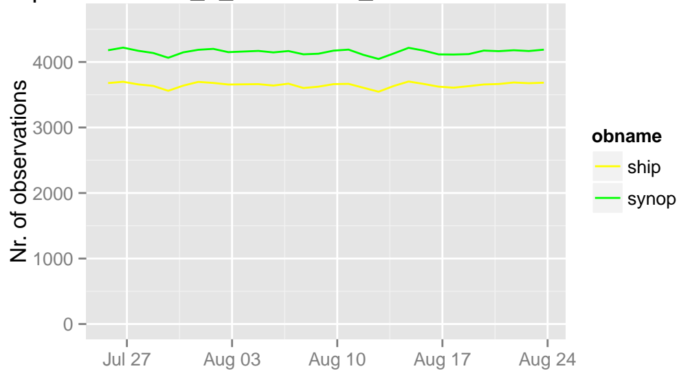
/opdata/arome2_5_main/ecma_sfc/ts/ecma.db 18 UTC
