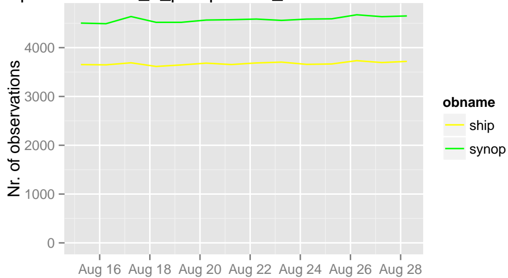
/opdata/arome2_5_preop/ecma_sfc/ts/ecma.db 06 UTC
