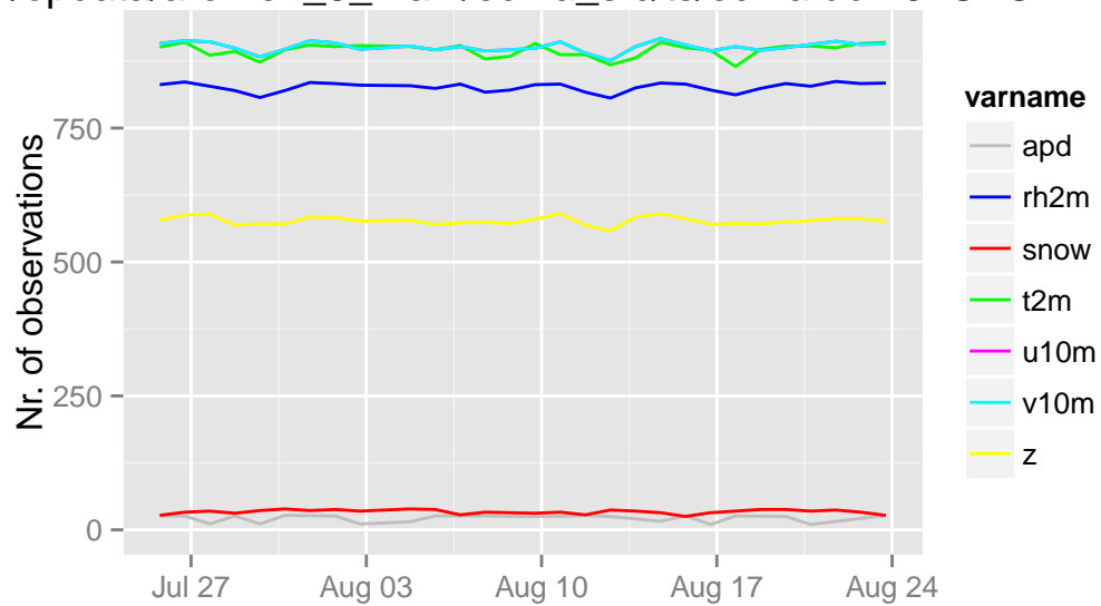
/opdata/arome2_5_main/ecma_sfc/ts/ecma.db 18 UTC
