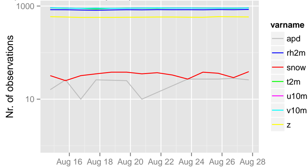
/opdata/arome2_5_preop/ecma_sfc/ts/ecma.db 18 UTC
