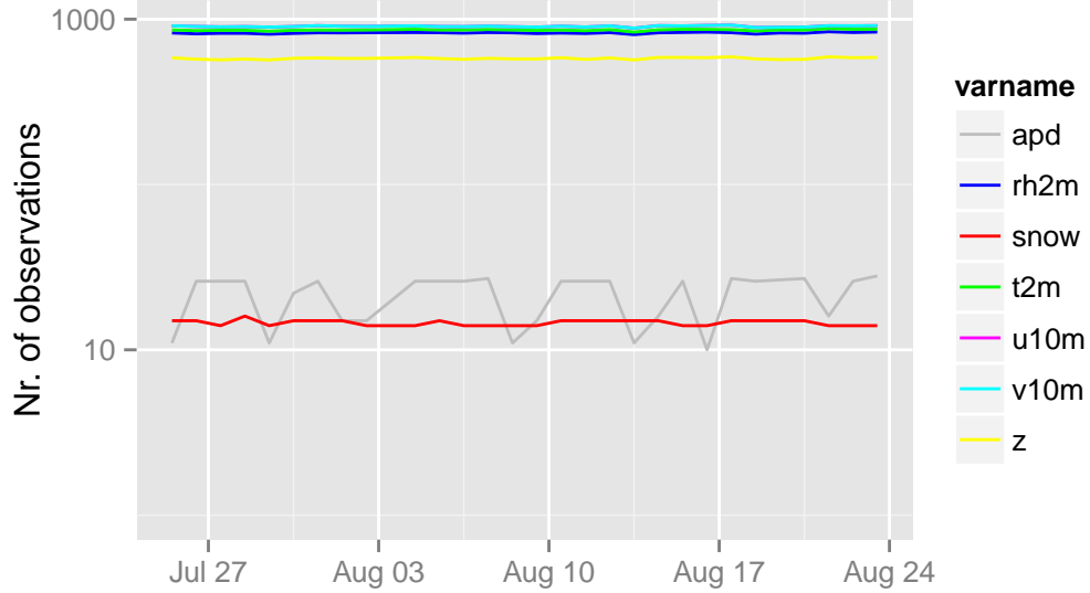
/opdata/arome2_5_main/ecma_sfc/ts/ecma.db 12 UTC
